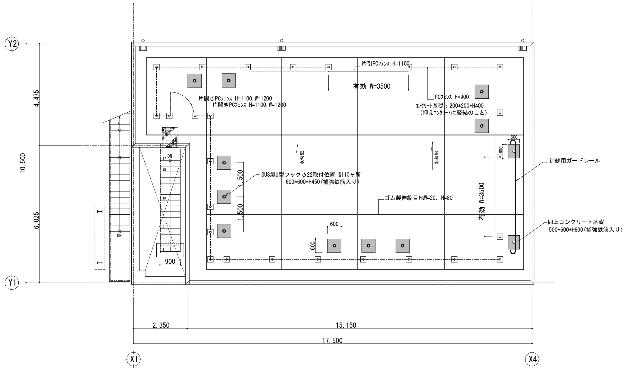
R階平面図 S=1/100
